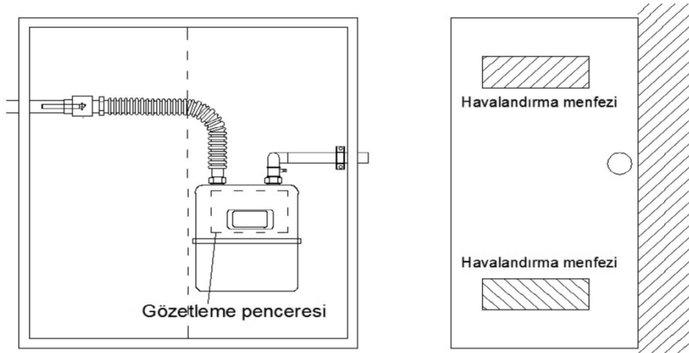
Şekil 17. Sayaç Kutusu
