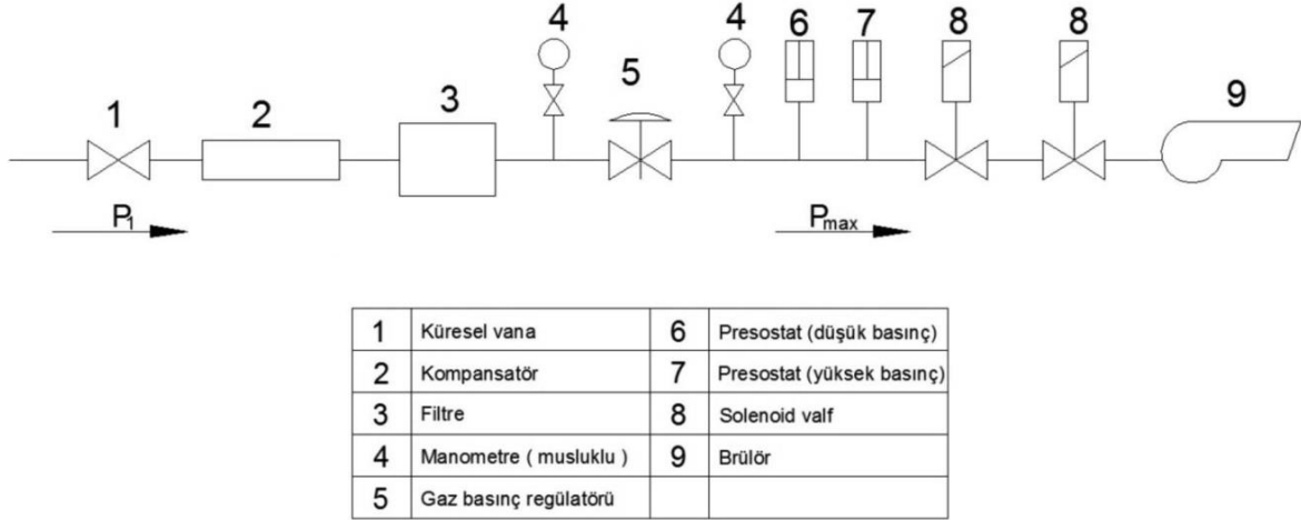
Şekil 40. Q_B < 1200 kW ve Düz Regülatör Kullanılması Durumunda Gaz Kontrol Hattı Ayrıntısı
