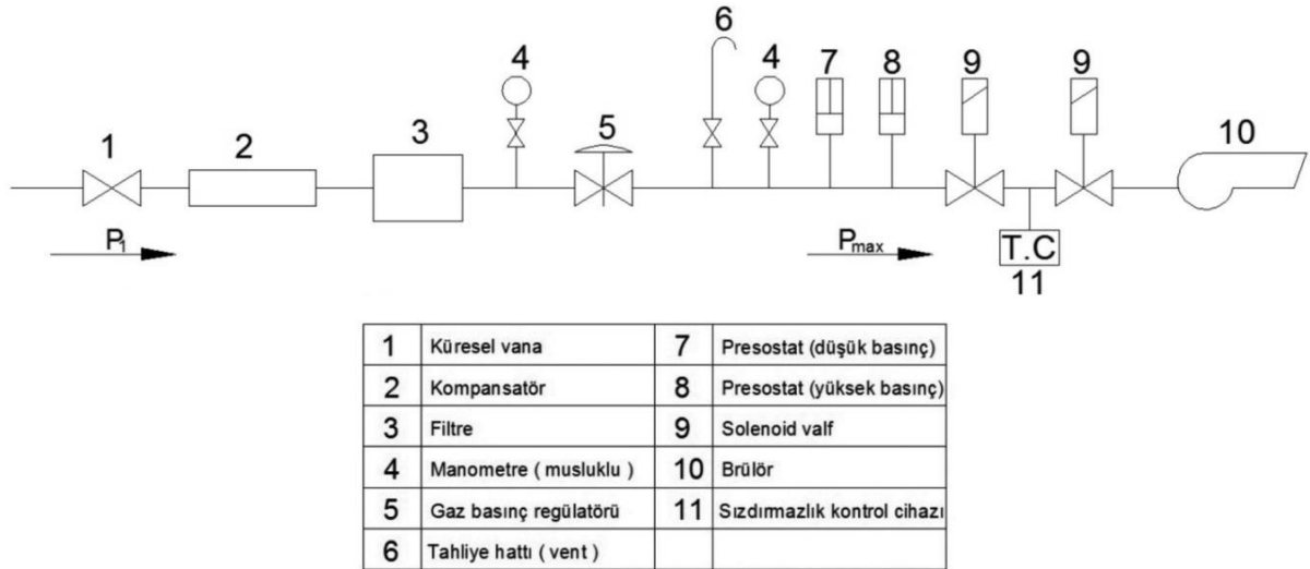
Şekil 41. Q_B \geq 1200 kW ve Düz Regülatör Kullanılması Durumunda Gaz Kontrol Hattı Ayrıntısı
