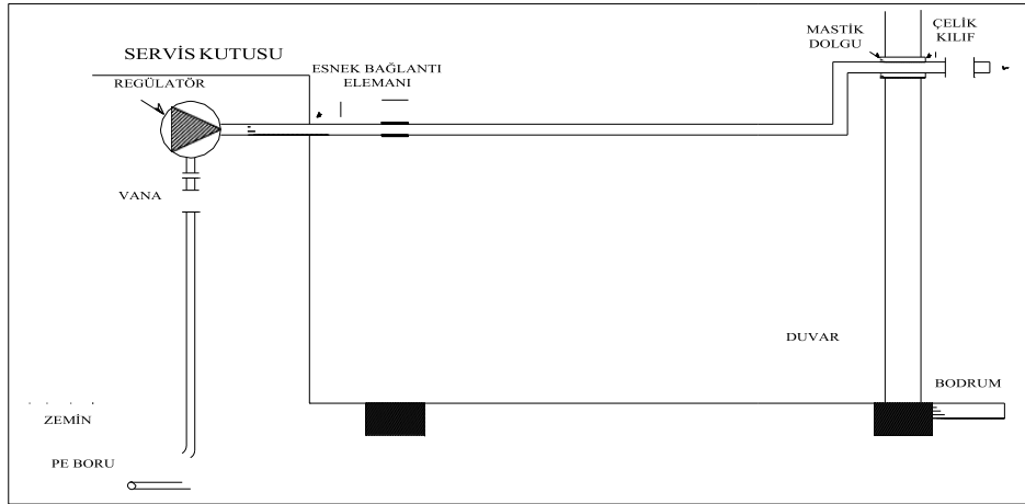
Şekil 1. Binalara Ait Servis Hatları Ve Servis Kutularının Yerleri, İşletmece Belirlendikten Sonra İç Tesisatın Bina Bağlantı Hatları
