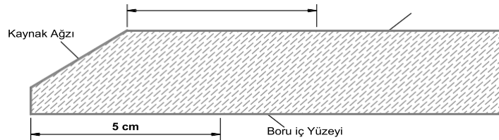
Şekil 3. Kaynak Ağzı
